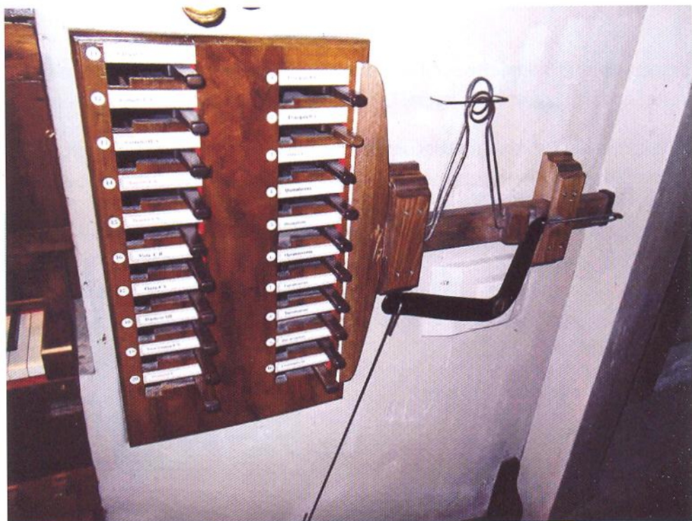
Tavola dei registri con meccanismo del Ripieno dopo il restauro
