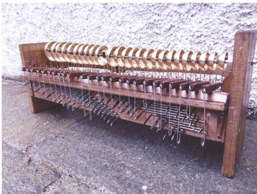
Campanelli con relativi martelli e meccanica
